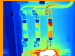
Fusibles calientes
