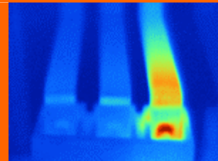
Conexión de barra colectora
